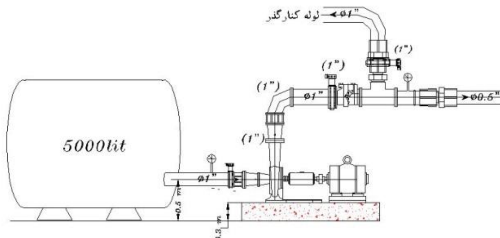
شکل ۱- نقشه شماتیک سیستم و لوله اجراء شده
