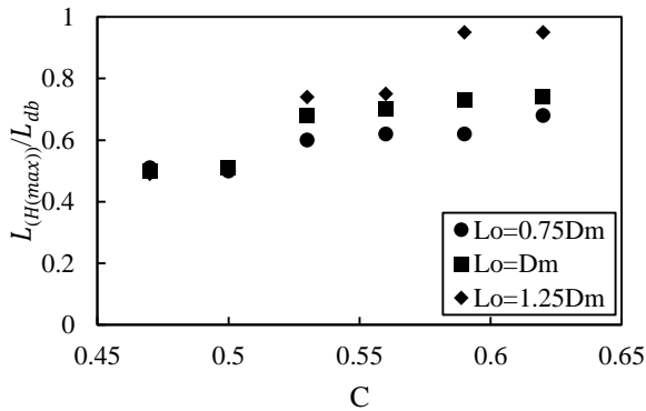
شکل ۷- رابطه بین پارامترهای بی‌بعد \frac{L_t}{L_{db}} ، \frac{L_{H(max)}}{L_{db}} و غلظت جریان واریزه‌ای، (الف) شیب فلوم ۵ درجه، (ب) شیب فلوم ۷ درجه و (ج) شیب فلوم ۹ درجه
