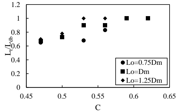
شکل ۷- رابطه بین پارامترهای بی‌بعد \frac{L_t}{L_{db}} ، \frac{L_{H(max)}}{L_{db}} و غلظت جریان واریزه‌ای، (الف) شیب فلوم ۵ درجه، (ب) شیب فلوم ۷ درجه و (ج) شیب فلوم ۹ درجه
