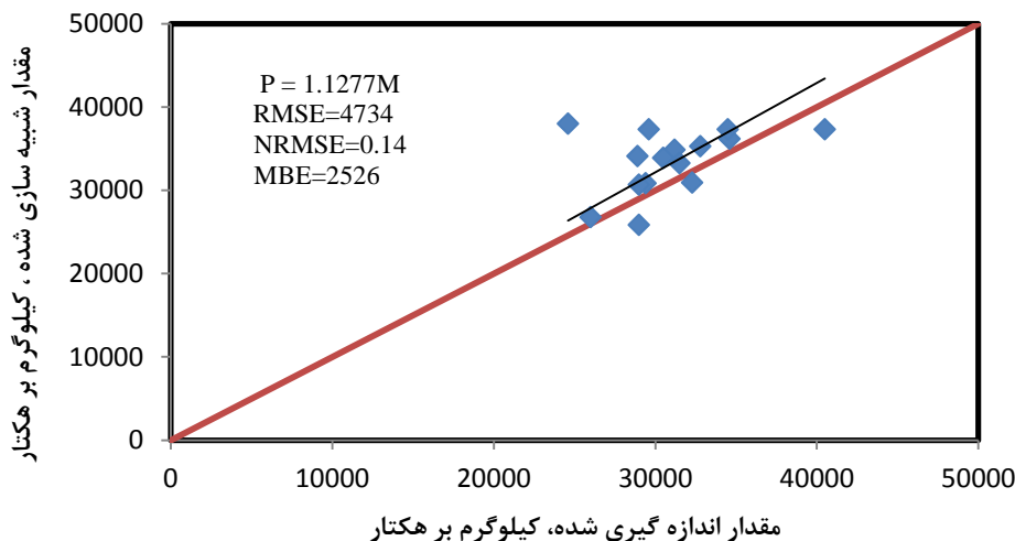
شکل ۶- مقایسه مقادیر شبیه سازی شده و اندازه گیری شده عملکرد سیب زمینی توسط روش تافته و همکاران (۲۰۱۳) و ضرایب واسنجی شده نسبت به خط یک به یک
