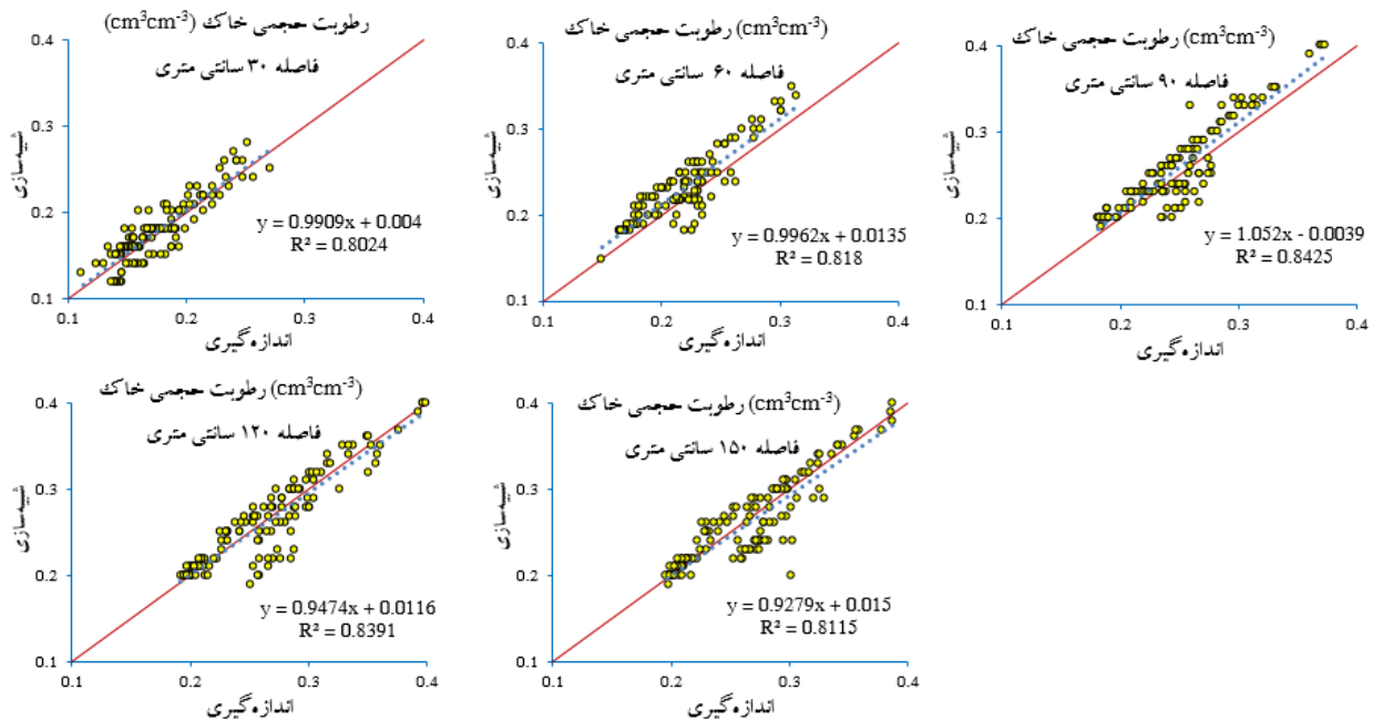
شکل ۵- ضریب تبیین ( R^2 ) رطوبت حجمی خاک مابین مقادیر اندازه‌گیری و شبیه‌سازی شده در فواصل شعاعی ۳۰، ۶۰، ۹۰، ۱۲۰، ۱۵۰ سانتی متری از تنه درخت
