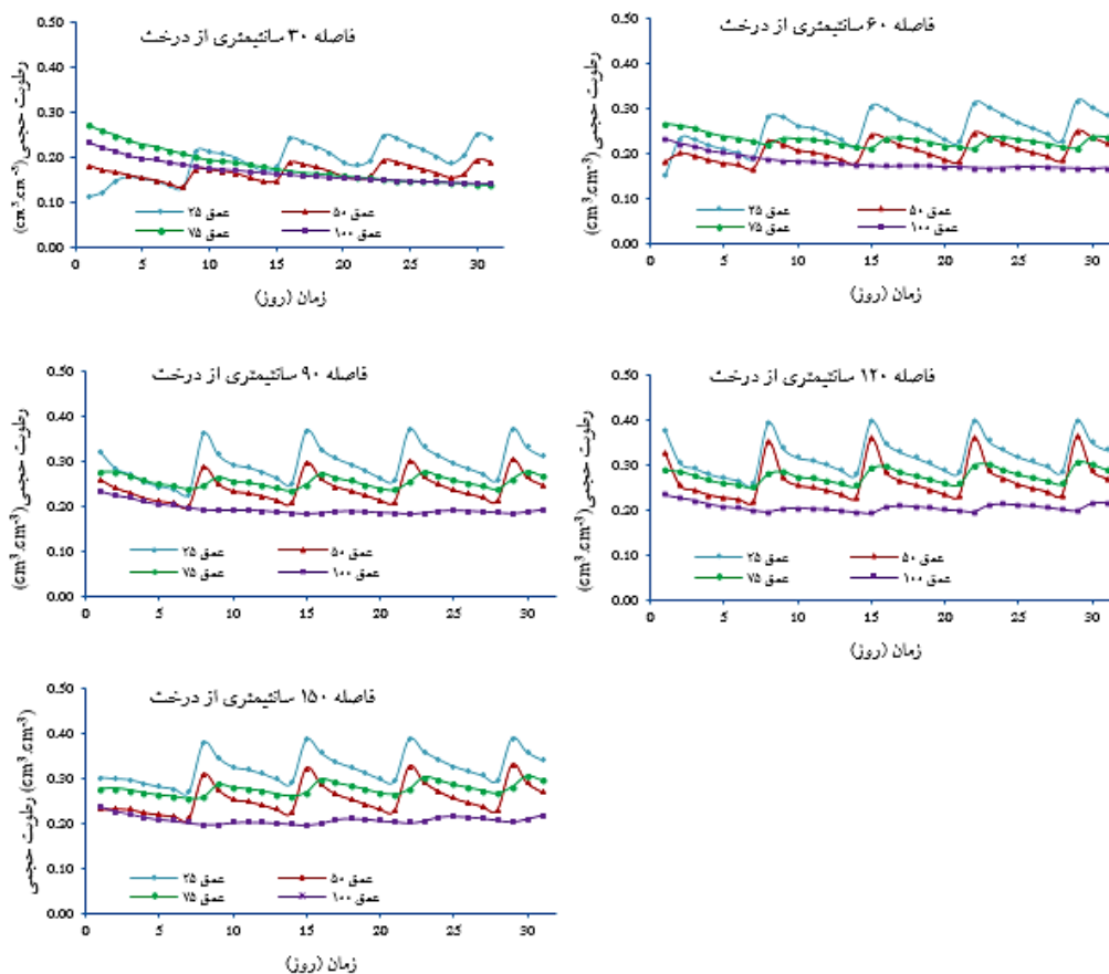
شکل ۳- رطوبت حجمی اندازه‌گیری شده ( \text{cm}^3.\text{cm}^{-3} ) توسط دستگاه TDR در چهار دور آبیاری در عمق‌های ۲۵، ۵۰، ۷۵ و ۱۰۰ سانتی متر در فواصل مختلف از تنه درخت
