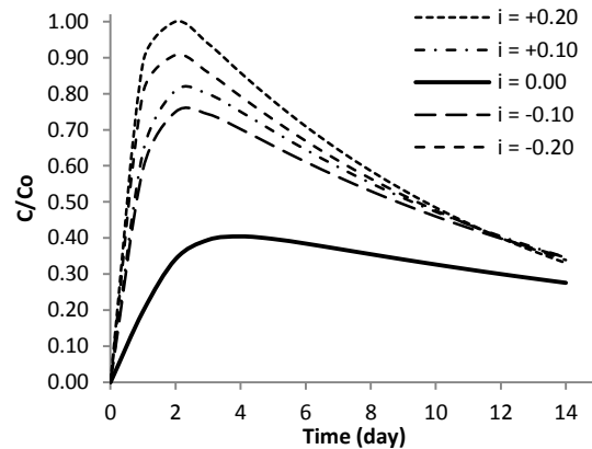
شکل ۱۰- تغییرات غلظت یون کلر در منبع پذیرنده در گرادیان‌های مختلف
