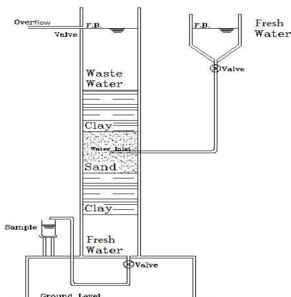
شکل ۱- تصویر شماتیک از نحوه‌ی اتصالات (آزمایش D-II)
