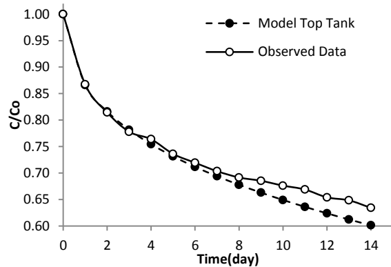
شکل ۵- مقایسه مدل و نتایج آزمایشگاهی در منبع آلاینده V-I
