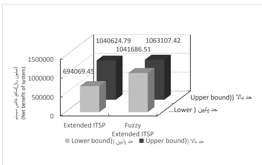
شکل ۴- مقایسه سود خالص حاصل از دو مدل ITSP توسعه داده شده و ITSP توسعه داده شده فازی در سد قلعه چای عجب شیر
