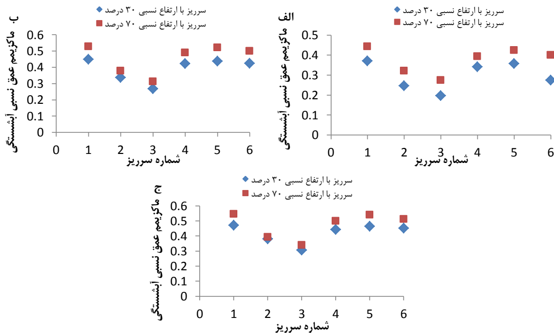
شکل ۱۱- ماکزیم عمق نسبی آبستتگی (ماکزیم عمق آبستتگی در دماغه سرریز نسبت به طول مؤثر سرریز) در دماغه سرریزها با ارتفاع‌های نسبی مختلف (ارتفاع سرریز نسبت به عمق آب ورودی) و شیب تاج صفر، الف: فرد ۳۵، ب: فرود ۳۹، ج: فرود ۴۳
