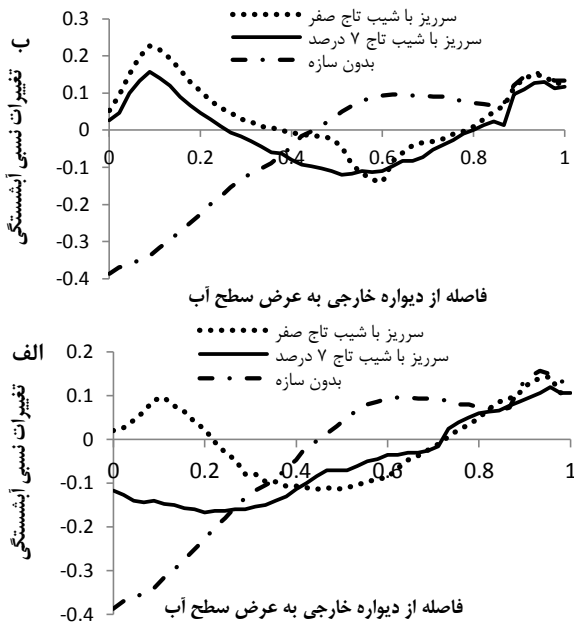
شکل ۸- اثر شیب تاج سرریزهای مستغرق بر تغییرات نسبی آبخستگی (تغییرات آبخستگی نسبت به طول مؤثر سرریز) در مقطع ۹۰ درجه با فرود 0/43+ ، الف: سرریز با ارتفاع ۳۰ درصد عمق آب ورودی، ب: سرریز با ارتفاع ۷۰ درصد عمق آب ورودی.
