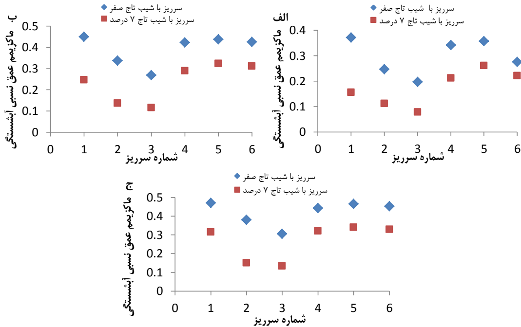
شکل ۱۲ - ماکزیمم عمق نسبی آبشستگی (ماکزیمم عمق آبشستگی در دماغه سرریز نسبت به طول مؤثر سرریز) در دماغه سرریزها با ارتفاع نسبی ۳۰ درصد عمق آب و رودی و شیب تاج متغیر، الف: فرود ۰/۳۵، ب: فرود ۰/۳۹ و ج: فرود ۰/۴۳
