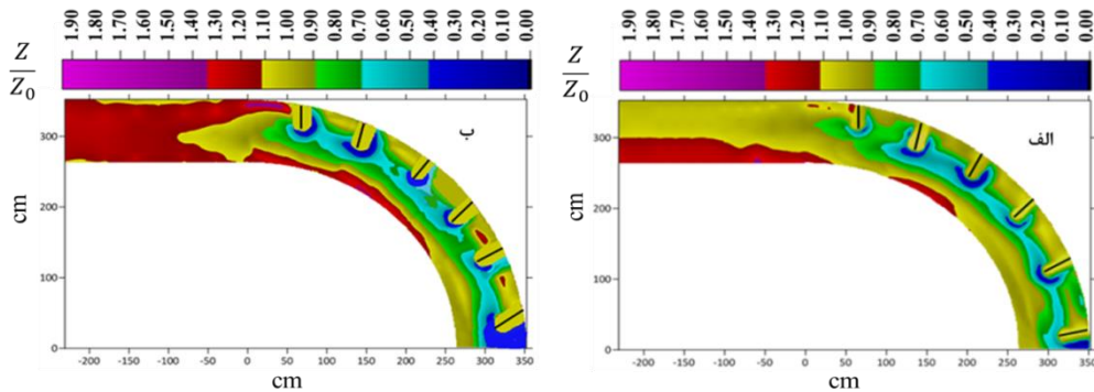
شکل ۵- تغییرات توپوگرافی بستر اطراف سرریزها با شیب تاج صفر ( Z ) نسبت به ضخامت بستر اولیه ( Z_0 )، الف: سرریز با ارتفاع نسبی ۳۰ درصد عمق آب ورودی، ب: سرریز با ارتفاع نسبی ۷۰ درصد عمق آب ورودی
