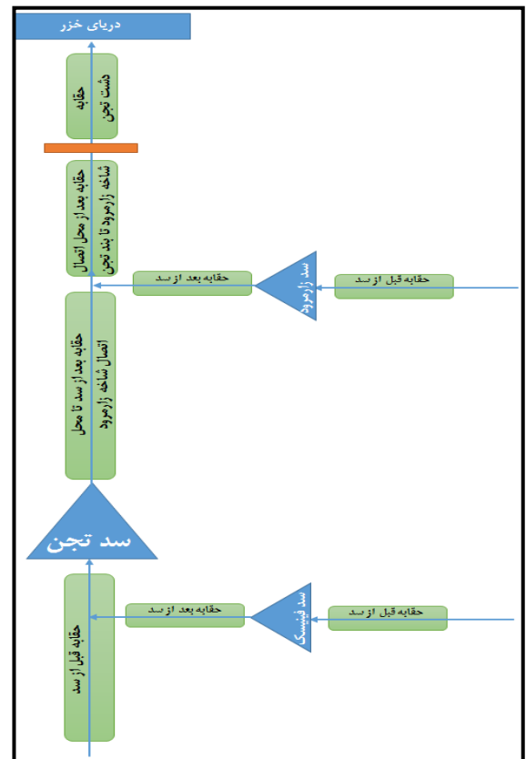
ب. شماتیک بازه‌های مصارف حوضه آبریز رودخانه تاجن
