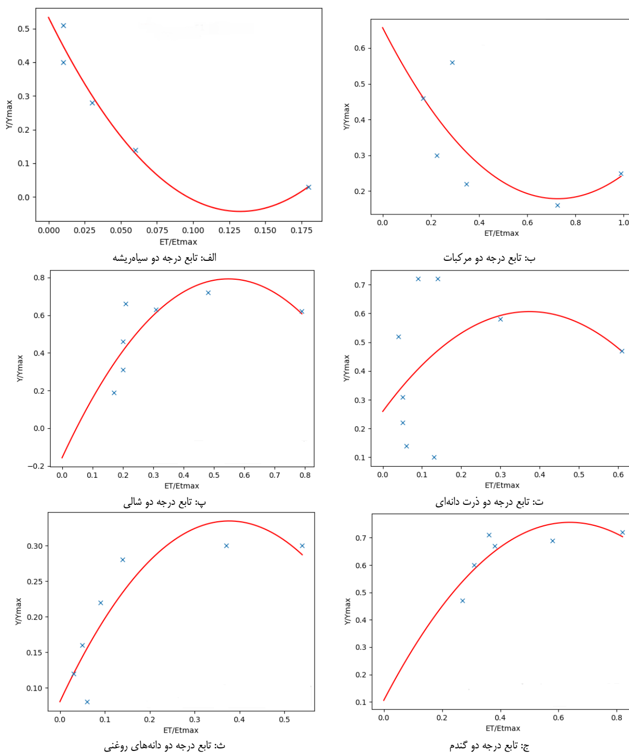
شکل ۵- نمودارهای انتخابی توابع عملکرد از مدل تلفیقی PySD-PCSE
