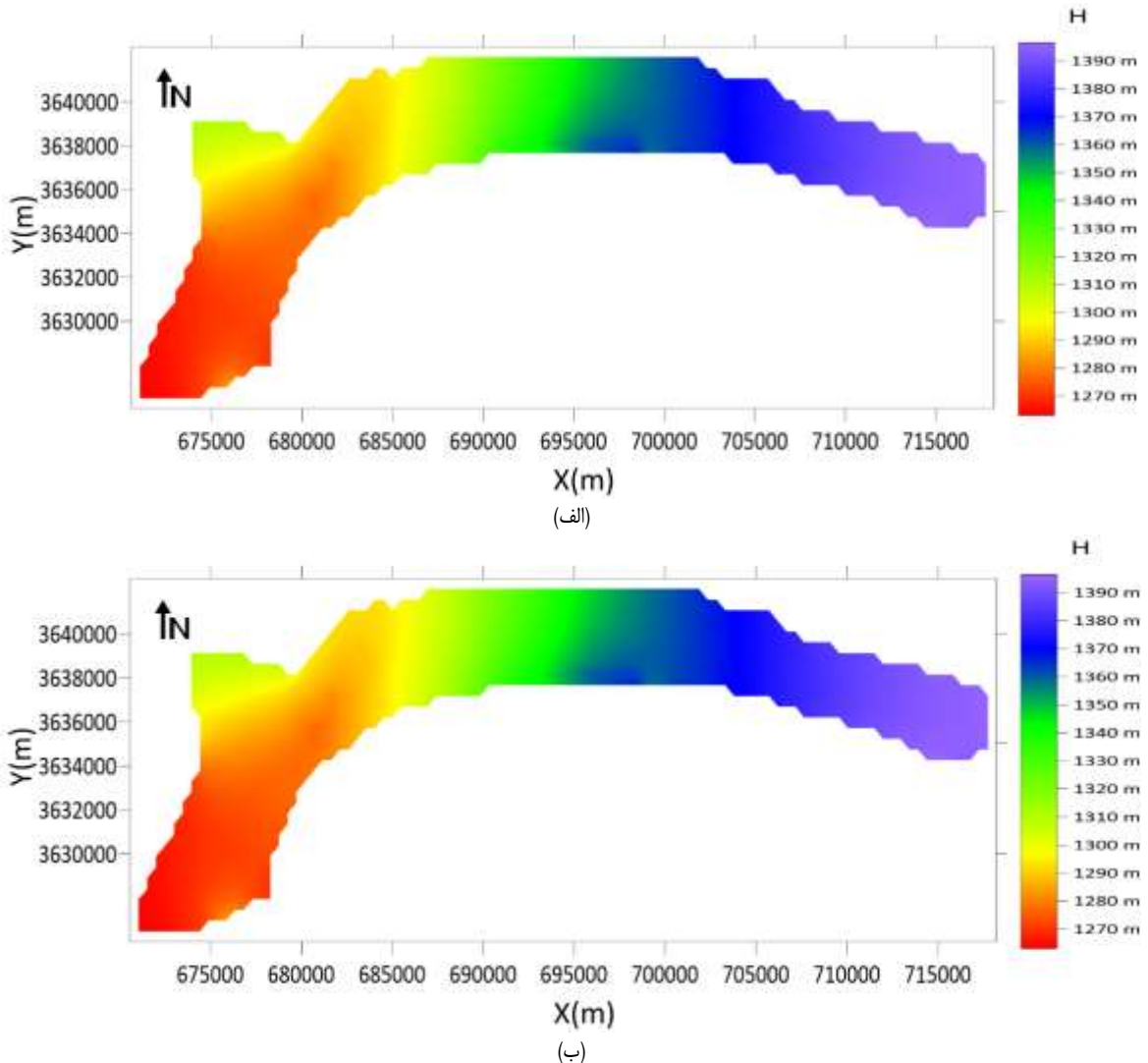
شکل ۶- الف) نتایج گرفته شده از روش بدون شبکه در حالت غیرماندگار در اول دوره. ب) نتایج گرفته شده از مدل به روش بدون شبکه در انتهای دوره (Mohtashami et al. 2019)
