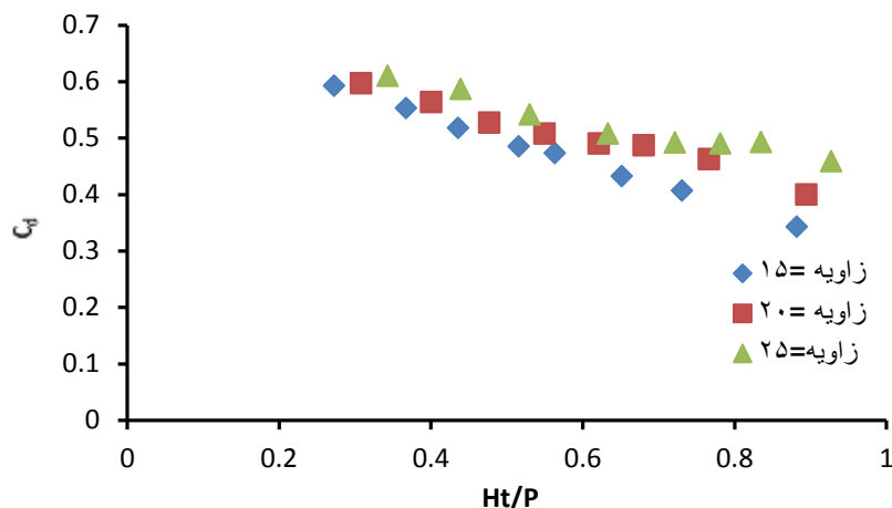
شکل ۳- مقایسه ضریب دبی مدل ترکیبی با زوایای مختلف برای بازشدگی درجه ۲ سانتی متر
