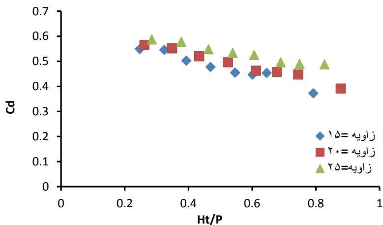
شکل ۵- مقایسه ضریب دبی مدل ترکیبی با زوایای مختلف برای بازشدگی درجه ۶ سانتی متر
