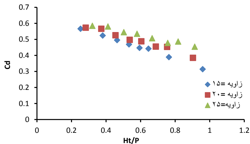
شکل ۴- مقایسه ضریب دبی مدل ترکیبی با زوایای مختلف برای بازشدگی درجه ۴ سانتی متر
