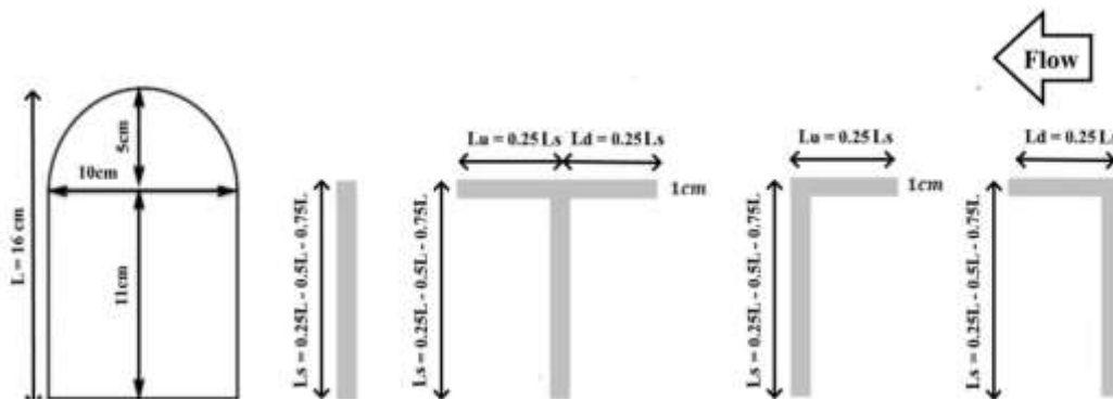
شکل ۴- ابعاد تکیه‌گاه و آبشکن‌های مورد استفاده در آزمایش‌ها
