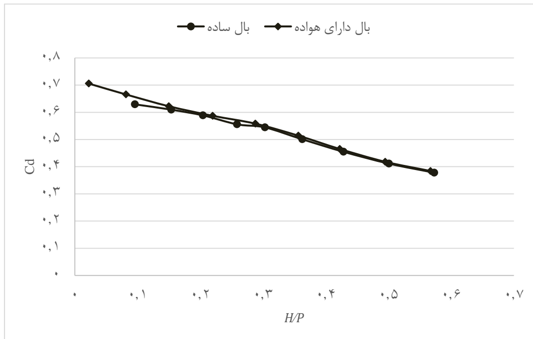
شکل ۱۲- تغییرات C_d بر حسب H/P در سرریز کنگره‌ای مثلثی با بال ساده بدون هواده و با هواده L/W = 4
