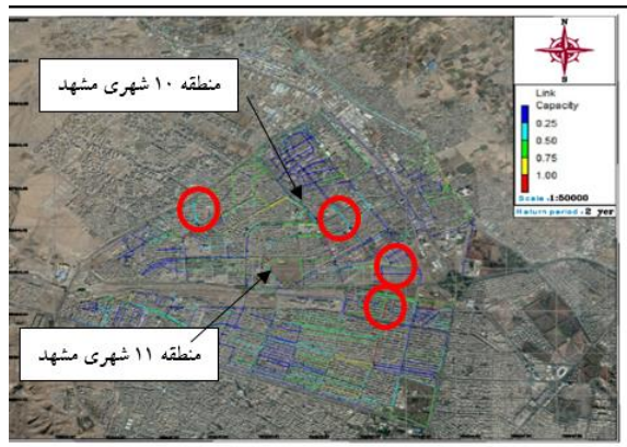
دوره بازگشت ۲ ساله
