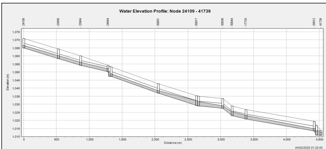
شکل ۱۰- عملکرد کانال امامیه- امام هادی در شرایط سیل با دوره بازگشت ۵۰ ساله
