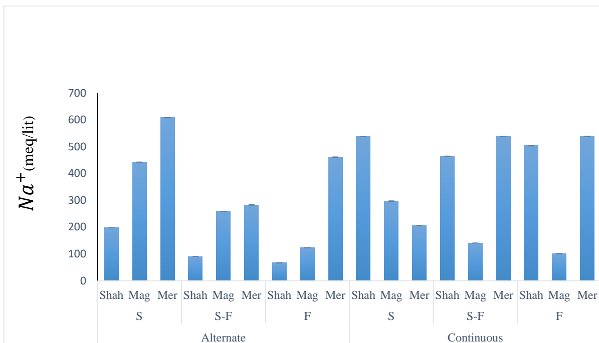
شکل ۷- تغییرات غلظت سدیم (Na + ) خروجی از زهاب حاصل از آبشویی خاک، در شکل بالا S نماد تیمار آب شور، F نماد تیمار آب شیرین و S-F نماد تیمار آب شور-شیرین می باشد. نماد Shah نماد تیمار شاهد، Mag نماد تیمار مگنت و Mer نماد تیمار رینگ مروس است و Alternate (روش متناوب) و Continuous (روش پیوسته) می باشد.
