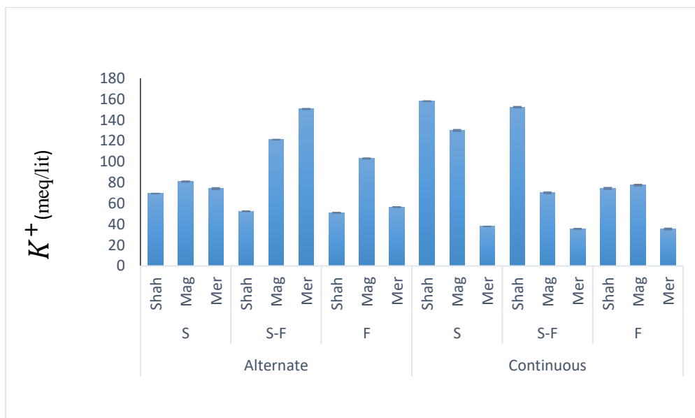
شکل ۸- تغییرات غلظت پتاسیم ( K^+ ) خروجی از زهاب حاصل از آبشویی خاک، در شکل بالا S نماد تیمار آب شور، F نماد تیمار آب شیرین، S-F نماد تیمار آب شور-شیرین می‌باشد و Shah نماد تیمار شاهد، Mag نماد تیمار مگنت، Mer نماد تیمار رینگ مروس است و Alternate (روش متناوب) و Continuous (روش دائم) می‌باشد.
