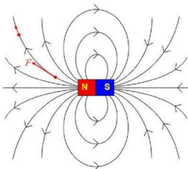
شکل -Error! No text of specified style in document. آرایش الکترون‌ها در میدان مغناطیسی
