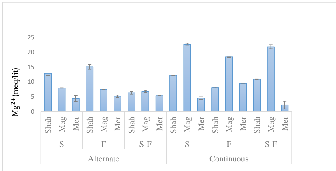
شکل ۱۰- تغییرات غلظت منیزیم خروجی در زهاب حاصل از آیشویی خاک، در شکل بالا S نماد تیمار آب شور، F نماد تیمار آب شیرین، S-، F نماد تیمار آب شور-شیرین می‌باشد و Shah نماد تیمار شاهد، Mag نماد تیمار مگنت، Mer نماد تیمار رینگ مروس است و Alternate (روش متناوب) و Continuous (روش دائم) می‌باشد.
