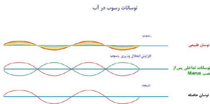
شکل ۶- نحوه ایجاد نوسانات رینگ مروس در آب
