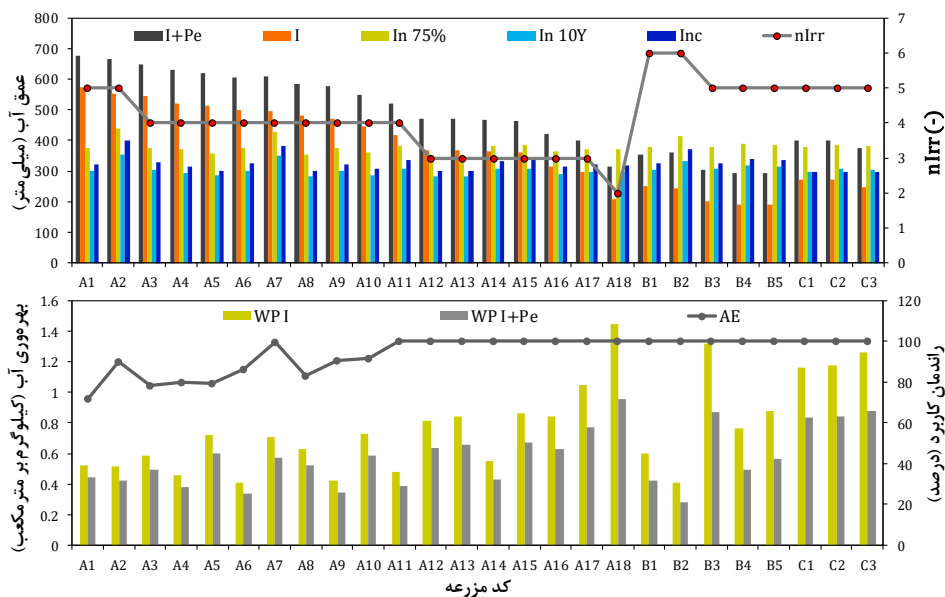
توضیحات: در این شکل، I و P به ترتیب، مقادیر فصلی آب کاربردی و بارش مؤثر، I_{n75\%} ، I_{n10Y} و I_{nc} به ترتیب، برآوردهای نیاز آبی خالص به‌ازای سطح احتمال وقوع ۷۵ درصد، میانگین ۱۰ سال اخیر و فصل زراعی مطالعاتی، nIrr و AE به ترتیب تعداد نوبت‌های آبیاری اعمال شده و راندمان کاربرد است. کدهای مزارع با حروف A، B و C به ترتیب، بیانگر مزارع با روش آبیاری شیاری، بارانی سنتریپوت و بارانی کلاسیک ثابت است.
