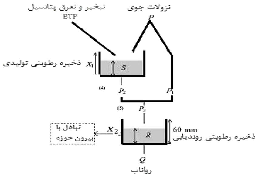
شکل ۳- دیاگرام مدل GR2M
