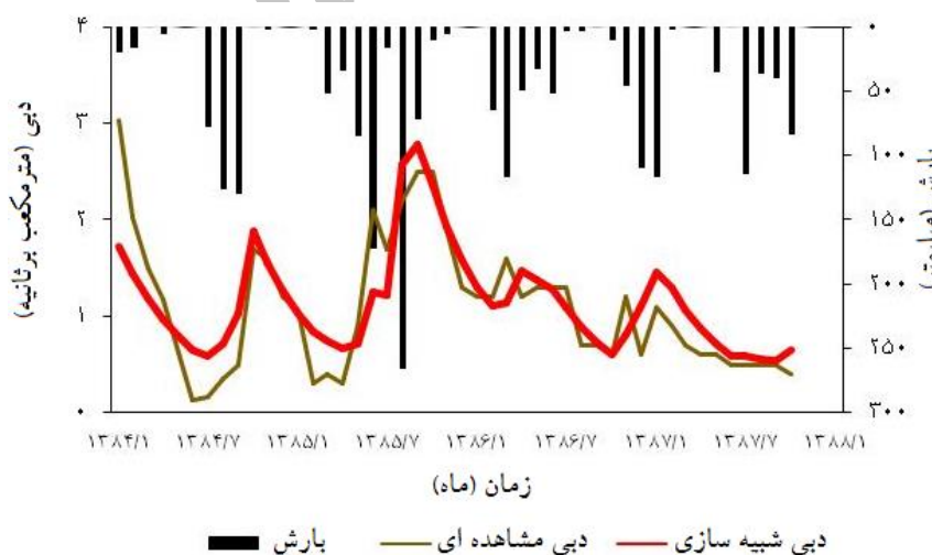
شکل ۵- نتایج مدل IHACRES برای شبیه سازی جریان ماهانه حوضه آبخیز دره تخت در مرحله اعتبارسنجی
