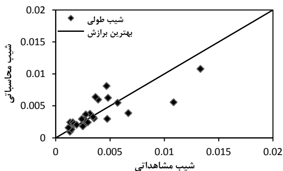
شکل ۵- مقایسه شیب طولی بستر مشاهداتی و محاسباتی
