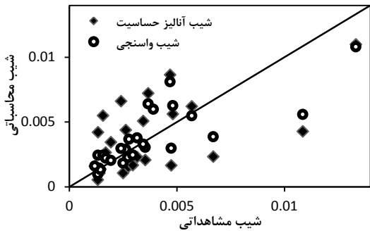
شکل ۱۳- آنالیز حساسیت اثر اندازه رسوب بر شیب
