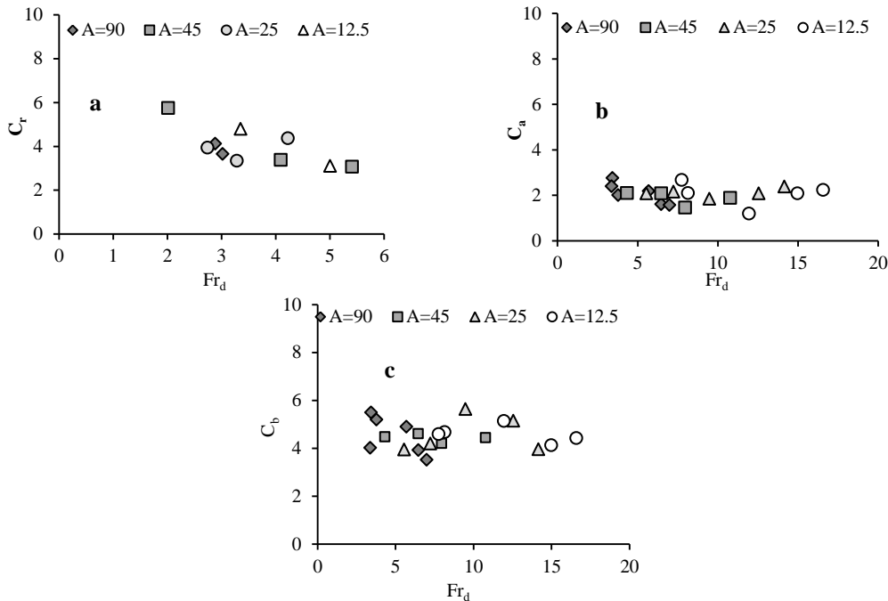
شکل ۷- (a) ضرایب انتشار جریان جت سطحی همگرا در مقابل عدد فرود چگال، الف) بدون شیب طولی، ب) دارای شیب طولی در راستای طول فلوم، c) دارای شیب طولی در راستای عرض فلوم
