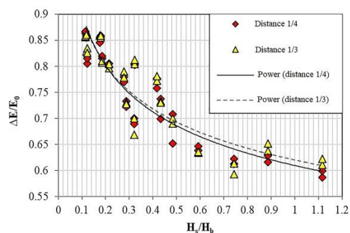
Fig. 8- Variation of flow dissipating energy against parameter H_s/H_b for different baffle's distances شکل ۸- تغییرات استهلاک انرژی در برابر پارامتر H_s/H_b برای فاصله‌ی متفاوت موانع
