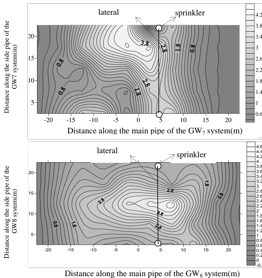
Fig. 3 - Water distribution pattern around adjacent tube tested by GW_7 and GW_8 irrigation systems شکل ۳- الگوی پخش آب در اطراف لوله جانبی مورد آزمایش سیستم‌های آبیاری GW_8 و GW_7
