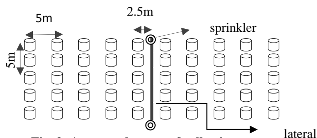
Fig. 2- Arrange the cans of collecting water شکل ۲- ترتیب قرار گرفتن قوطی‌های جمع‌آوری آب
