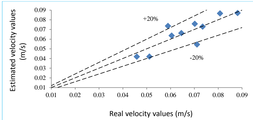
Fig.12- Results of density current head velocity modeling in separation point شکل ۱۲- نتایج حاصل از مدل سازی سرعت پیشانی جریان غلیظ در نقطه جدشدگی
