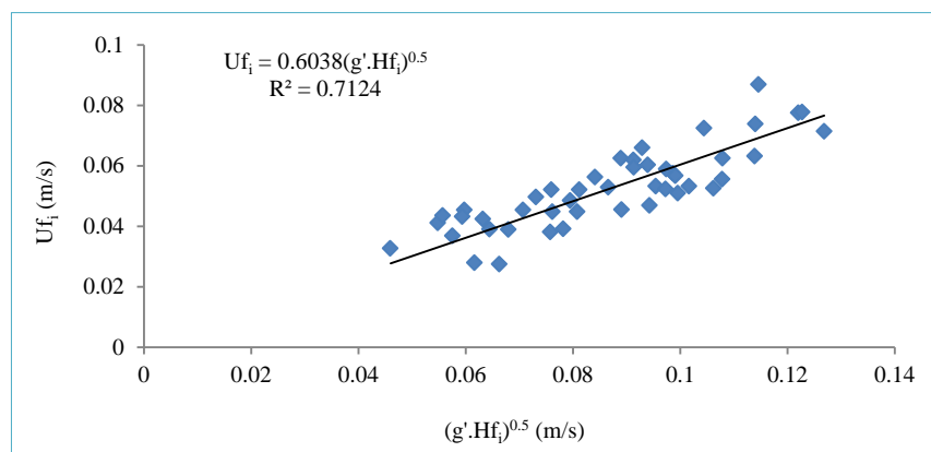
Fig.14- Variations of U_{fi} versus (g'.hfi)^{0.5} in initial part of interflow density current شکل ۱۴- تغییرات U_{fi} در مقابل (g'.hfi)^{0.5} در قسمت ابتدایی جریان غلیظ میانگذر
