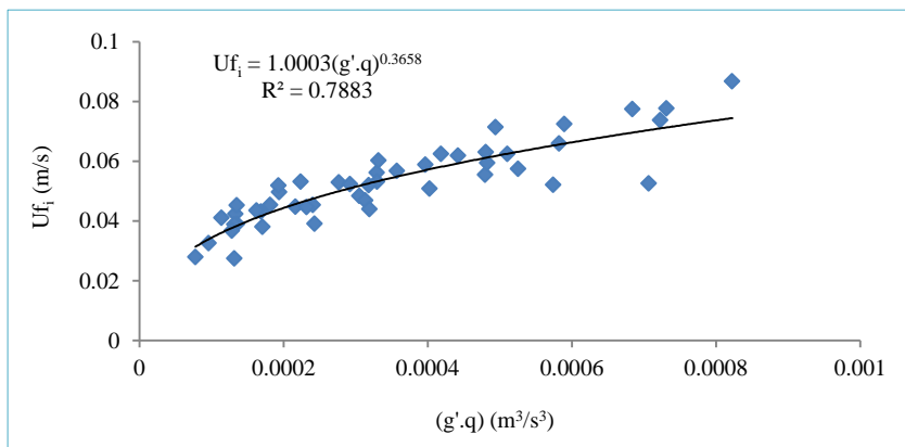
Fig. 13- Variations of head velocity in initial of interflow density current versus buoyancy flux شکل ۱۳- تغییرات سرعت پیشانی در ابتدای جریان غلیظ میانگذر در مقابل فلاکس شناوری
