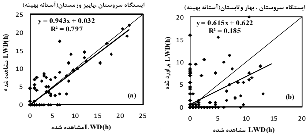
شکل ۳- رابطه بین LWD اندازه‌گیری شده و برآورد شده توسط مدل آستانه رطوبتی با آستانه بهینه، (a) آستانه ۸۱٪، (b) آستانه ۶۸٪
