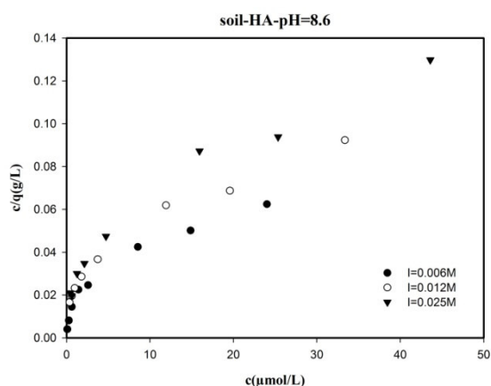
شکل ۸. برازش معادله لنگموئیر یک مکانی بر داده های جذبی در اسید هیومیک خاکی در \text{pH} برابر ۸٫۶
