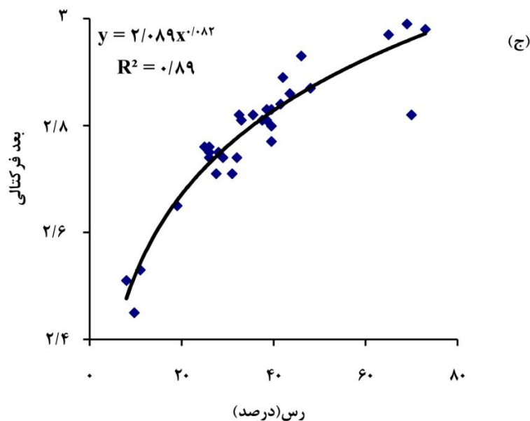
شکل ۱. رابطه بعد فرکتالی با درصد شن (الف)، درصد سیلت (ب) و درصد رس (ج)
