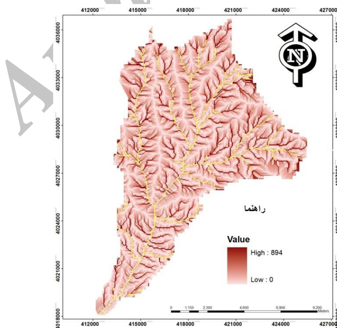
شکل ۳. نقشه پتانسیل فرسایش حوضه آبخیز باراجین
