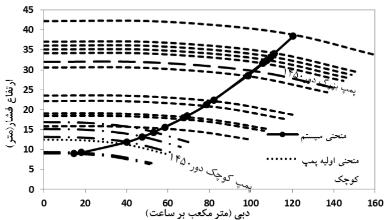
شکل ۲. منحنی پمپ و سیستم در دورهای مختلف پمپ‌های دور متغیر
