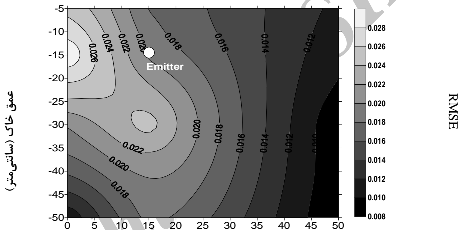
شکل ۳. توزیع خطای RMSE در مرحله صحت‌سنجی برای سراسر مدت شبیه‌سازی فاصله (سانتی‌متر) عمق خاک (سانتی‌متر)
