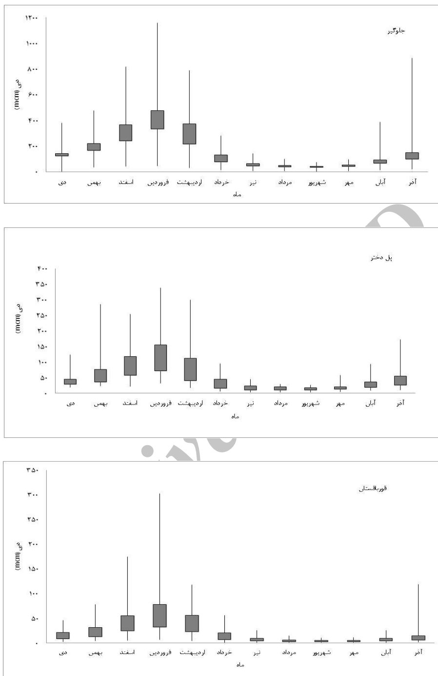
شکل ۴. منحنی توزیع دبی برای احتمالات ۲۵ و ۷۵ درصد در ایستگاه‌های آب‌سنجی جولوگیر، پل دختر و قورباقستان در حوضه کرخه
