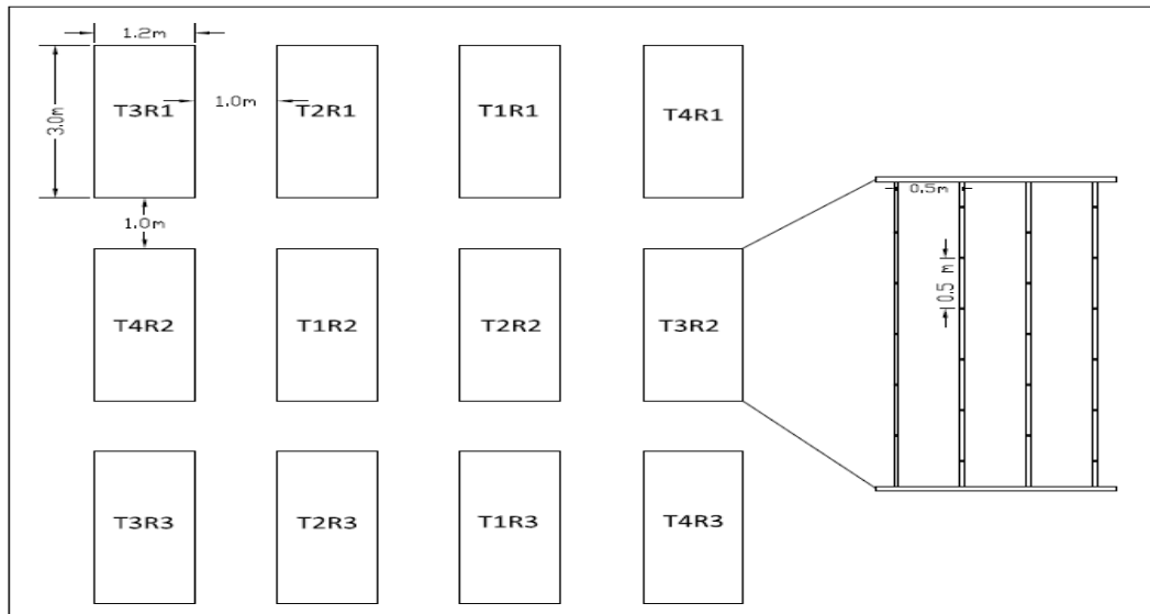
شکل ۱. نمای طرح آزمایشی و محل قرارگیری لوله ها در کرت های آزمایشی
