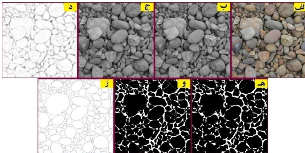
شکل ۵- مراحل پردازش تصویر: الف) تعیین خط مقیاس در تصویر رنگی برش داده شده، ب) تصویر خاکستری هشت‌بیتی، ج) تصویر پس از عبور دادن از فیلتر Median، د) تصویر پس از اعمال عملگر حذف پس‌زمینه، ه) ایجاد نواحی حدی (تصویر باینری)، و) اعمال عملگر Watershedding و ز) برازش بیضی‌ها بر ذرات
