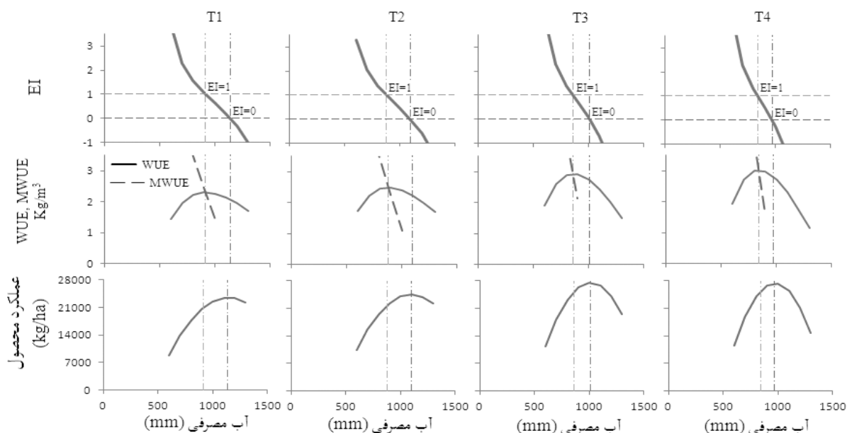
شکل ۲- منحنی تغییرات Y , WUE, MWUE, EI و برای تیمارهای اصلی T1 الی T4
