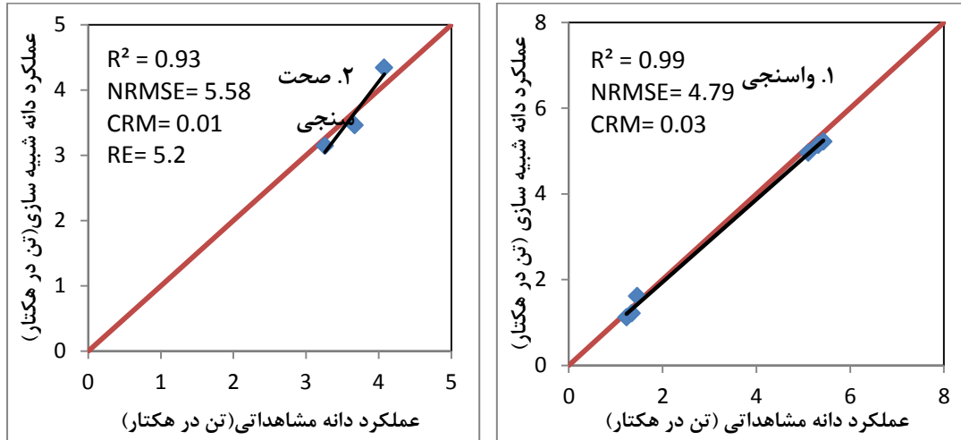
شکل ۳- همبستگی بین مقادیر مشاهداتی و شبیه‌سازی عملکرد دانه
