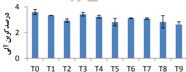
شکل ۳. میانگین درصد کربن آلی و انحراف معیار آن در خاک پس از تابش مایکروویو در تیمارهای مختلف آزمایشی تاگوچی (T1-T9) و تیمار شاهد (T0)
