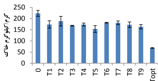
شکل ۲. میانگین غلظت هیدروکربن‌ها و انحراف معیار آن در خاک پس از تابش مایکروویو در تیمارهای مختلف آزمایشی تاگوچی (T1-T9). تیمار شاهد (T0) و در شرایط بهینه به دست آمده از آزمون‌های تاگوچی (Top).
