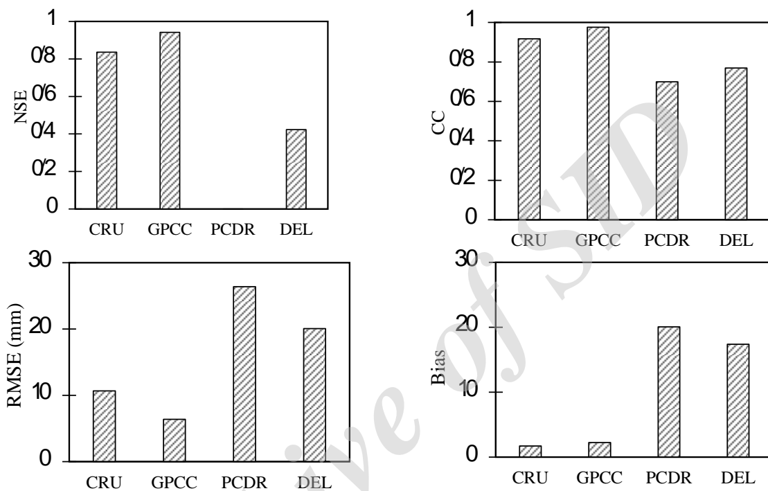
شکل ۴. تغییرات معیارهای کارایی ماهانه در حوضه ارومیه
