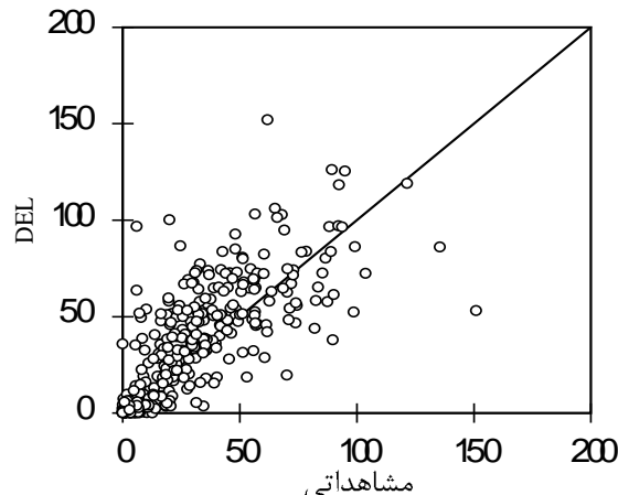
شکل ۳. میانگین بارش ماهانه مشاهداتی و پایگاه‌های جهانی در حوضه ارومیه
