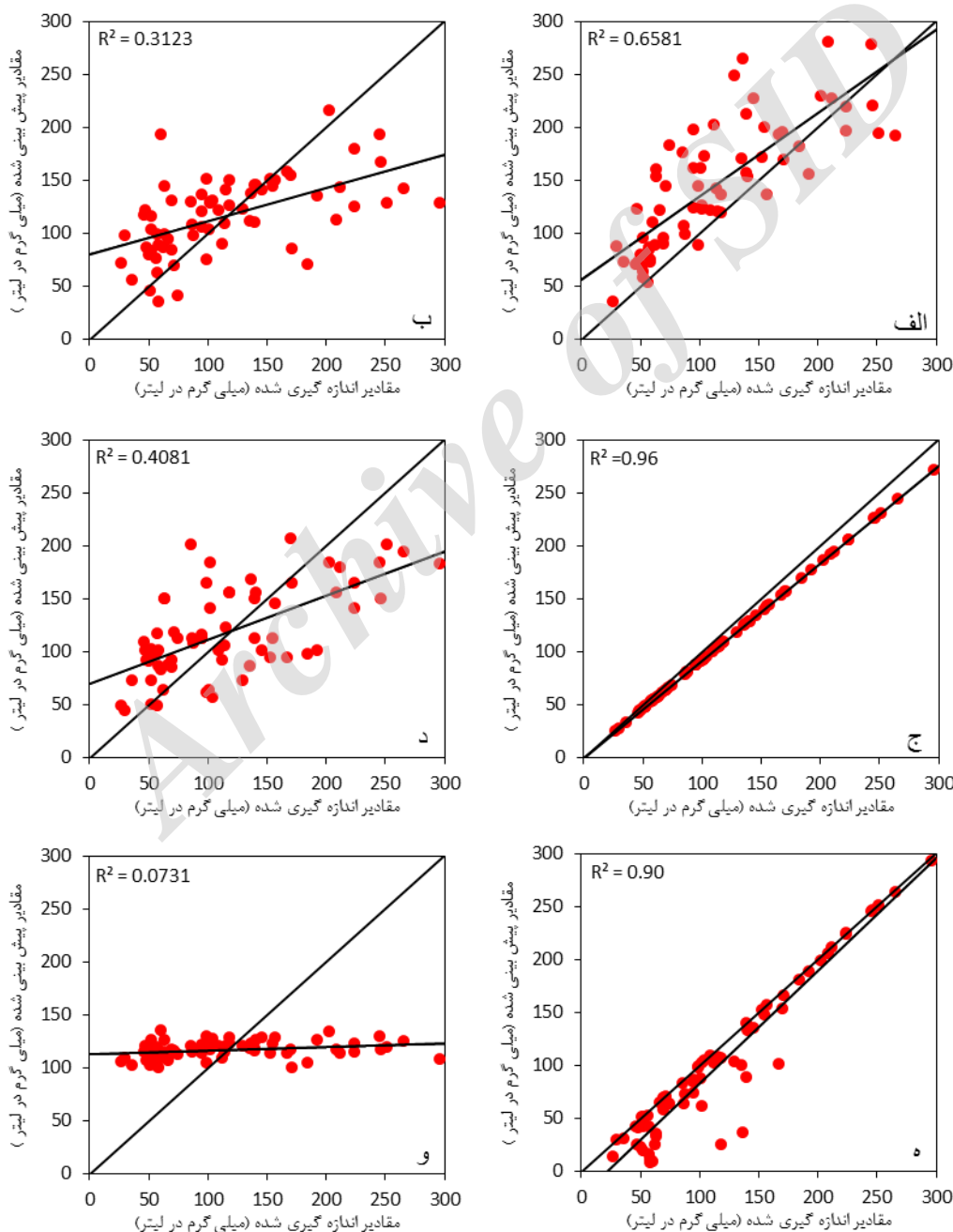
شکل ۳. نمودار پراکندگی مقادیر مشاهده شده و پیش‌بینی شده رسوب متوسط توسط مدل‌های الف: شبکه عصبی مصنوعی، ب: رگرسیون خطی، ج: فرآیند گوسی، د: k نزدیک‌ترین همسایه، ه: ماشین بردار پشتیبان تکاملی و و: ماشین بردار پشتیبان
