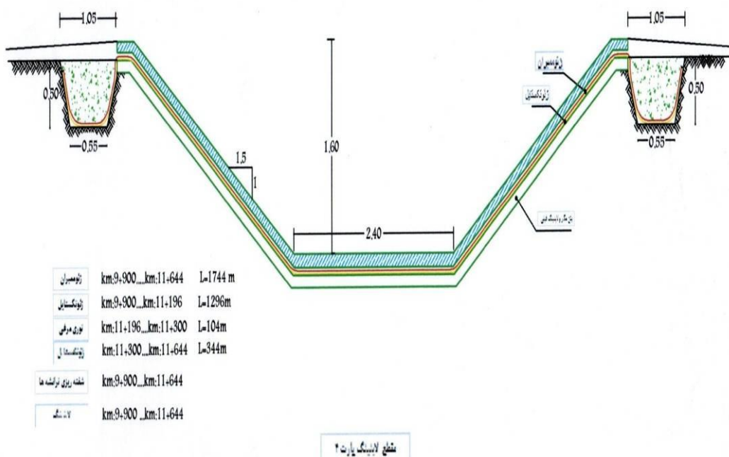
شکل ۲. مقاطع لایه‌بندی ژئوممبران کانال پمپاژ ۳ در منطقه مغان
