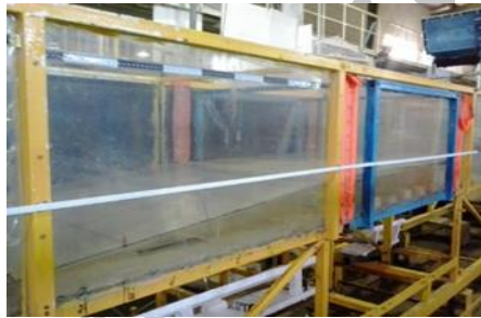
شکل ۳- نمای از مدل تاج پوشش کمربند سبز ساحلی و مدل شیب ساحل
