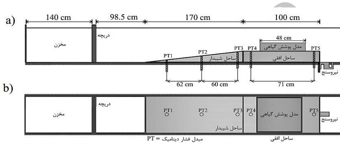
شکل ۲- به ترتیب (a) نمای از مقطع فلوم مستطیل شکل، و (b) نمای از پلان فلوم مستطیل شکل
