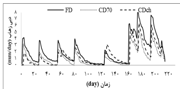
شکل ۶. هیدروگراف زهکشی در طول مدت کشت گندم
