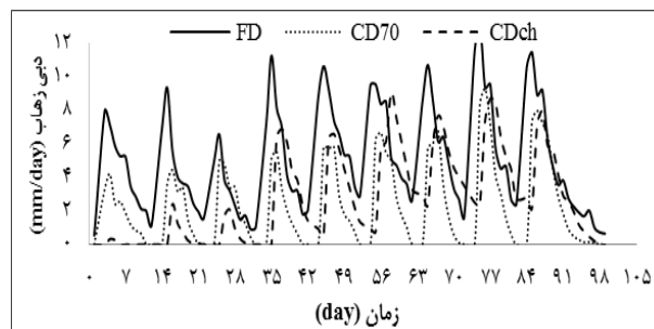
شکل ۵. هیدروگراف زهکشی در طول مدت کشت ذرت
