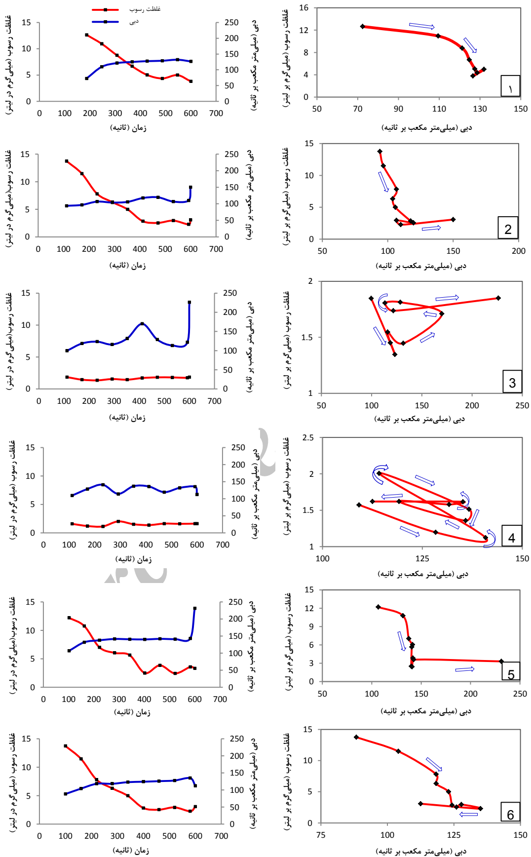
شکل ۳. آب نمود و رسوب نمود و حلقه های سنجه رسوبی شش رگبار پیاپی در شیب ۵ درصد و شدت ۹۰ میلی متر بر ساعت
