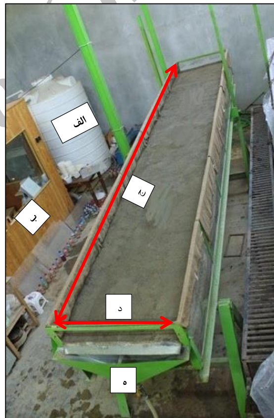
شکل ۱. تصویری از داخل شبیه‌ساز باران و فرسایش خاک: الف) مخزن تأمین آب باران، ب) اتاق کنترل، ج) طول پلات (۶ متر)، د) عرض پلات (۱ متر) و ه) سرریز (محل خروج رواناب و رسوب)
