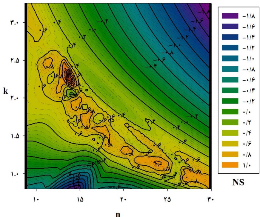
شکل ۷. مقادیر پارامتر n و k با عملکرد متفاوت در شبیه‌سازی هیدروگراف واحد بر اساس معیار ضریب کارایی
