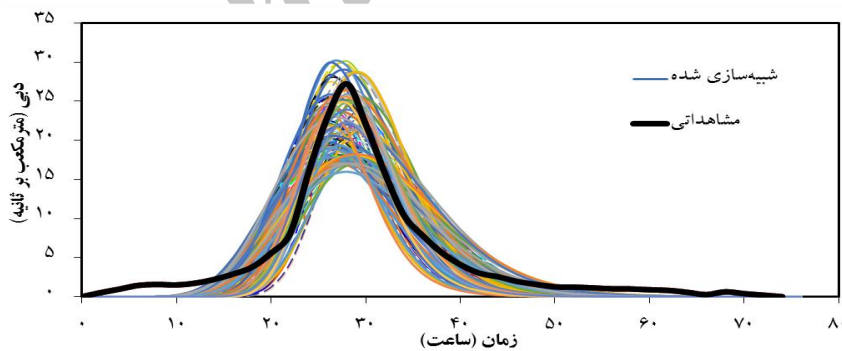
شکل ۲. هیدروگراف واحد مشاهداتی و شبیه‌سازی شده با مدل نش در حوضه آبخیز جعفرآباد
