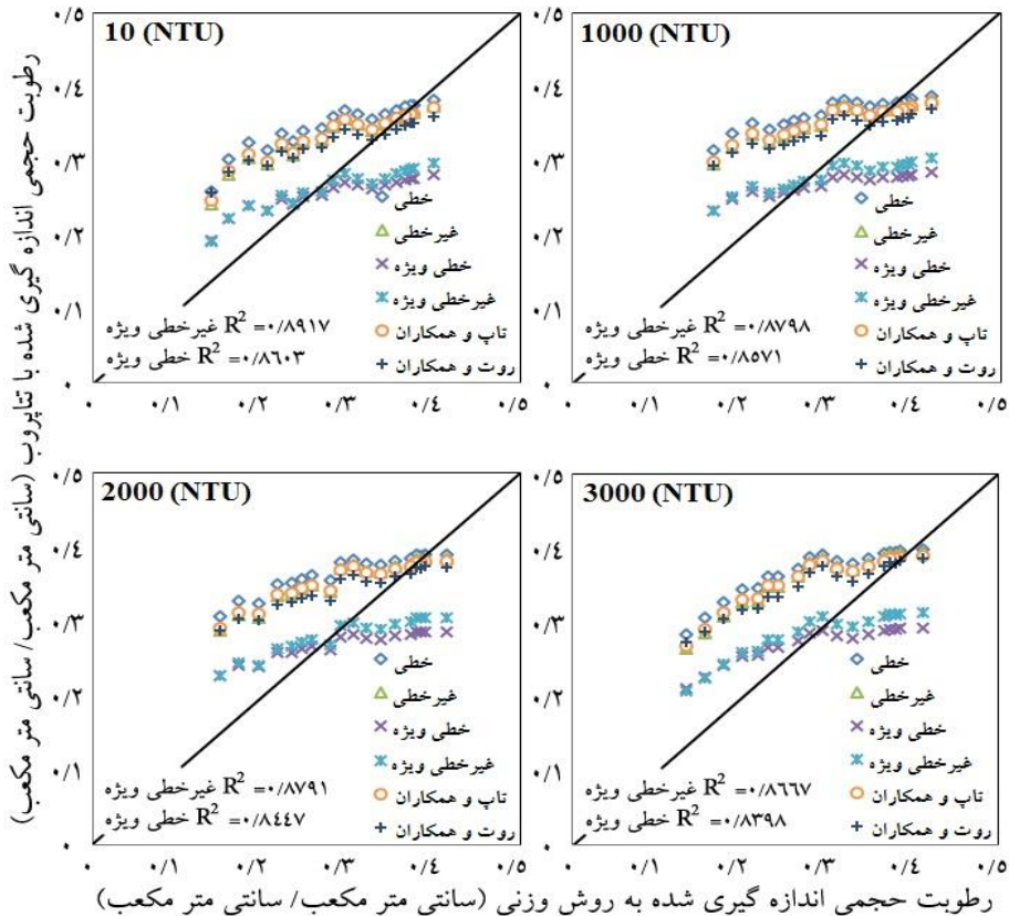
شکل ۲. مقایسه‌ی مقادیر رطوبت اندازه‌گیری شده به روش وزنی با مقادیر رطوبت اندازه‌گیری شده با دستگاه تترپروب در بافت لوم سیلینی تحت میزان مختلف کدورت.
