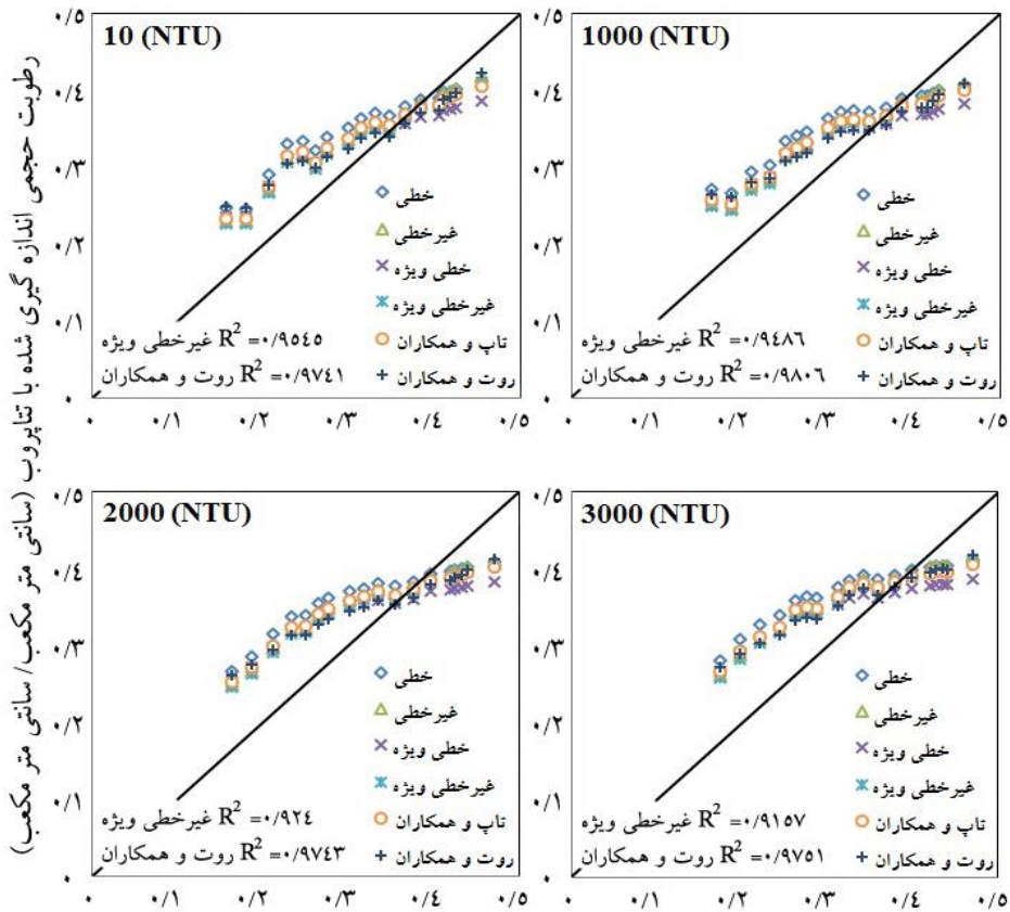
شکل ۱. مقایسه‌ی مقادیر رطوبت اندازه‌گیری شده به روش وزنی با مقادیر رطوبت اندازه‌گیری شده با دستگاه تترپروب در بافت لوم سیلینی تحت میزان مختلف کدورت.
