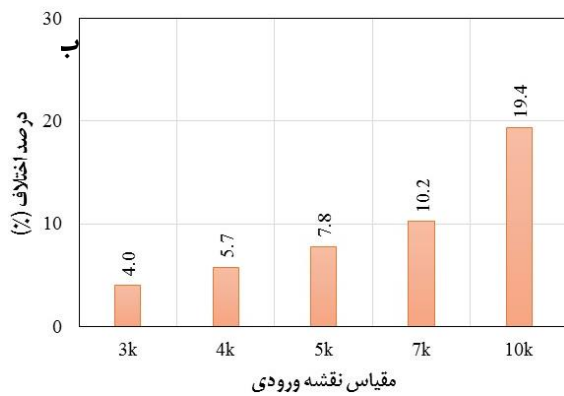
شکل ۴. میزان اختلاف بین پهنه سیلاب شبیه‌سازی در مقیاس‌های مختلف نسبت به نقشه مبنا (الف) سجاجس رود (ب) سرباز
