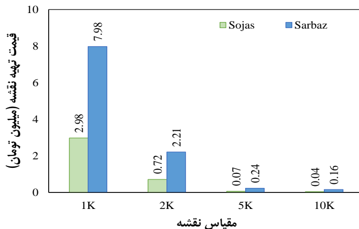
شکل ۷. هزینه موردنیاز برای تهیه یک کیلومتر نقشه با مقیاس‌های مختلف در رودخانه‌های سرباز و سجاجس رود درصد می‌رسد.
