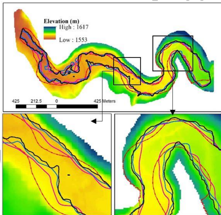
شکل ۵. تأثیر مقیاس نقشه بر پهنه سیلاب (رودخانه سجاجس رود)
