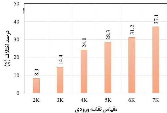
شکل ۴. میزان اختلاف بین پهنه سیلاب شبیه‌سازی در مقیاس‌های مختلف نسبت به نقشه مبنا (الف) سجاجس رود (ب) سرباز
