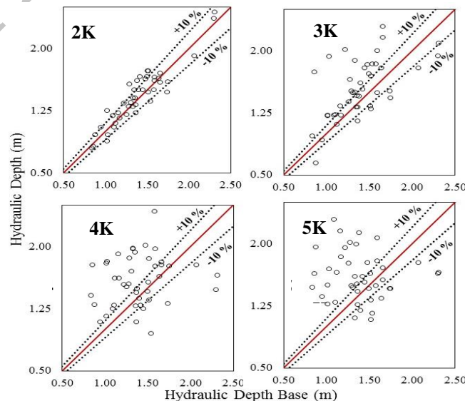
شکل ۶. تأثیر مقیاس نقشه بر عمق هیدرولیکی جریان در مقاطع عرضی مختلف (الف) رودخانه سرباز، (ب) رودخانه سجاس‌رود
