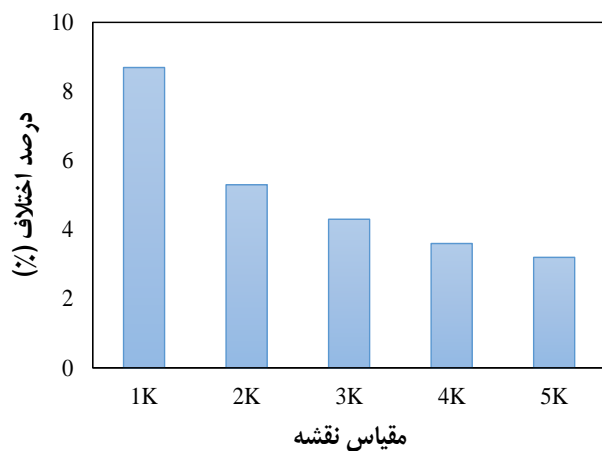
شکل ۸. اثر مقیاس نقشه توپوگرافی بر میزان اختلاف مدل‌های یک‌بعدی و دوبعدی در برآورد پهنه سیلاب (رودخانه سجاجس رود)
