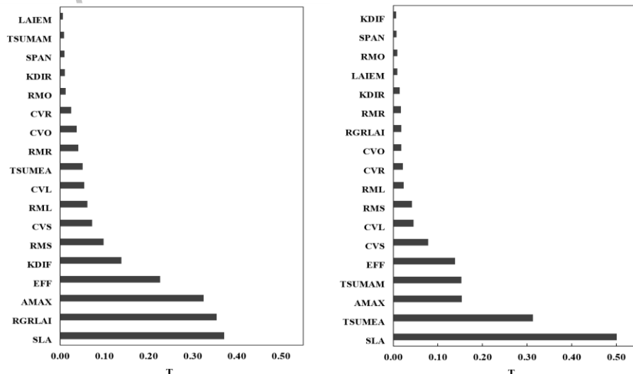
شکل ۲. مقایسه حساسیت پارامترهای گیاهی ذرت (راست) و گندم (چپ)
