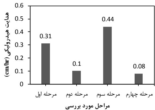
شکل ۴- مقادیر بهینه‌سازی شده هدایت هیدرولیکی در مراحل مختلف شبیه‌سازی
