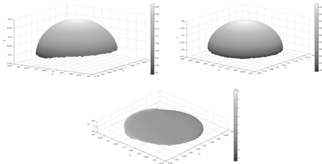
شکل ۱۰- (راست) مدل واقعی از تک گوی (کره)، (چپ) مدل رقومی تک گوی به روش SFM، (پایین) اختلاف نتایج مدل رقومی تک گوی به روش SFM با مدل واقعی
