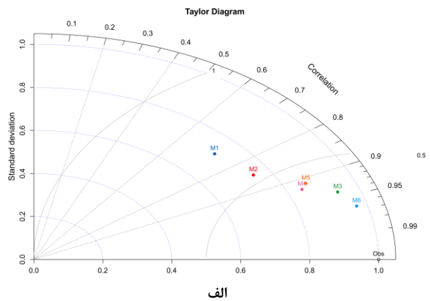
شکل ۷. دیاگرام تیلور شش مدل ترکیبی تولیدشده برای جریان ورودی به سدهای الف) بختيار ب) رودبار لرستان
