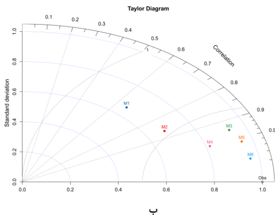
شکل ۷. دیاگرام تیلور شش مدل ترکیبی تولیدشده برای جریان ورودی به سدهای الف) بختيار ب) رودبار لرستان
