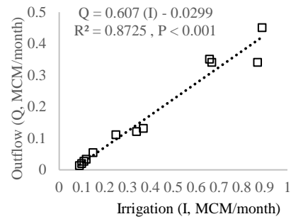
شکل ۴. رابطه و معادله رگرسیون خطی بین جریان خروجی ماهانه اندازه‌گیری شده در خروجی و آبیاری کاربردی ماهانه در شبکه طی فصول آبیاری ۸۸-۱۳۸۵
