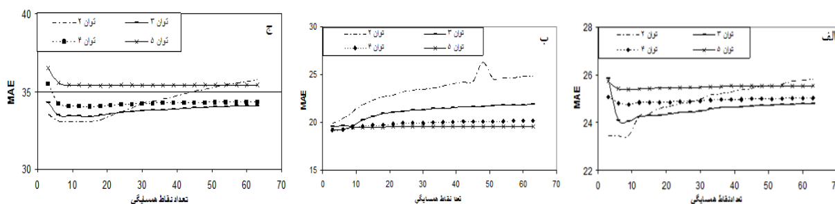
شکل ۳: ارزیابی تعداد نقاط همسایگی بهینه برای سال‌های آبی الف) ۷۶-۷۷، ب) ۶۸-۶۹، ج) ۷۱-۷۲ بر اساس MAE
