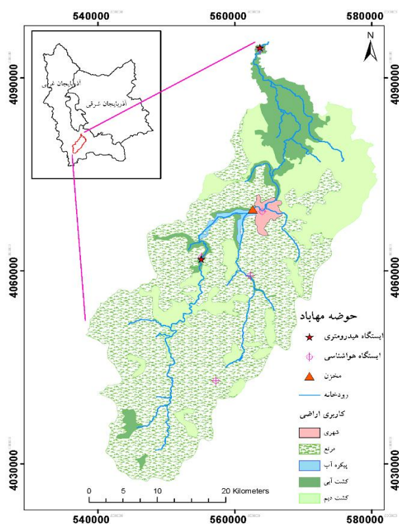
شکل ۱. موقعیت حوضه آبریز مهاباد
