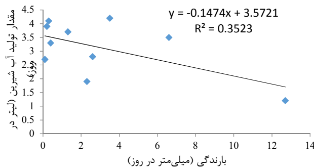
شکل ۸. مقدار تولید آب شیرین تقطیرگرهای خورشیدی گلخانه تحت تأثیر میانگین روزانه بارندگی (در روزهای بارانی)
