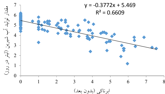
شکل ۶. مقدار تولید آب شیرین تقطیرگرهای خورشیدی گلخانه تحت تأثیر میانگین روزانه ابرنای
